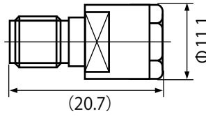
RP・SMA-J-316/U
