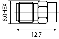
RP・SMA-J-316/U
